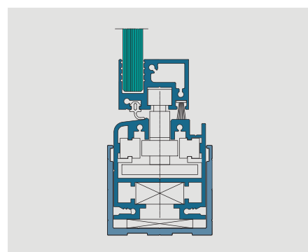
Vertikalschnitt mit Ausgleichsprofil unten Ausgleich bis 15 mm möglich
