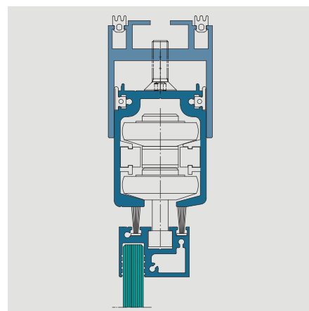
Vertikalschnitt mit Ausgleichsprofil oben Ausgleich bis 15 mm möglich
